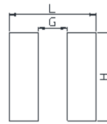
Land Pattern (Unit:mm)
