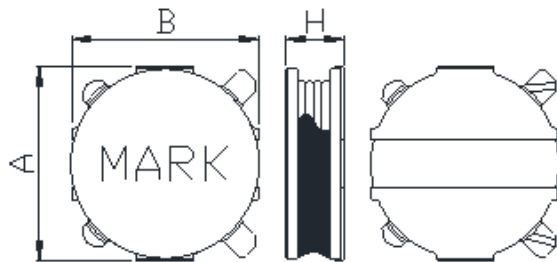
Dimension (Unit:mm)
