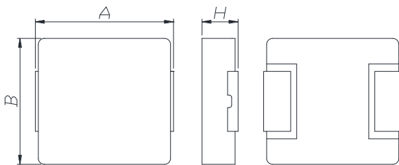
Dimension (Unit:mm)
