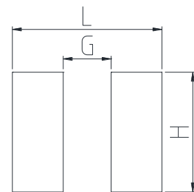
Land Pattern (Unit:mm)
