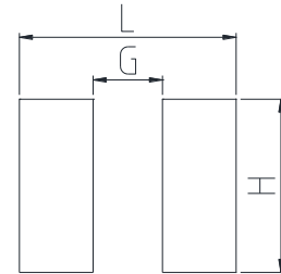
Land Pattern (Unit:mm)
