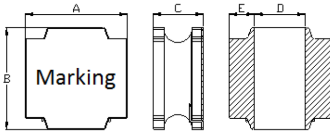
Dimension (Unit:mm)
