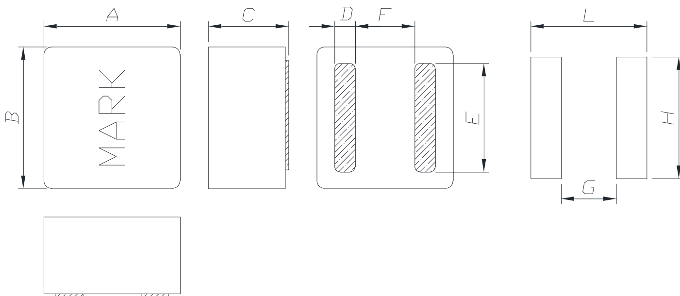
Dimension (Unit:mm)
