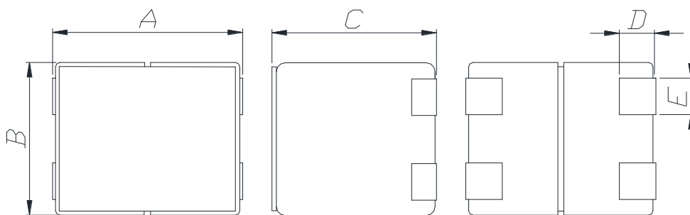
Dimension (Unit:mm)
