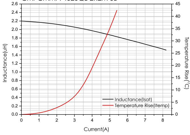
CMI-CMMPF4020QL-2R2M-SB
