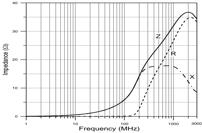
CME-NMCB160808H-070
