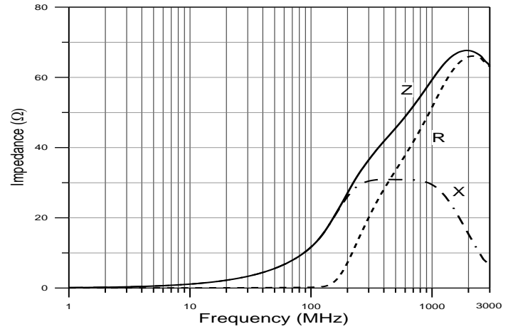
CME- NMCB160808H-100
