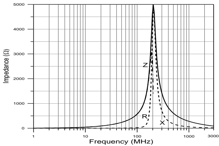
CME- NMCB160808H-601
