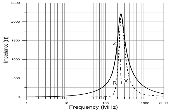
CME- NMCB160808H-301
