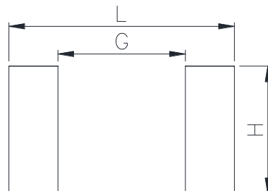
ランドパターン (単位: mm)
