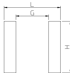
ランドパターン（単位：mm）
