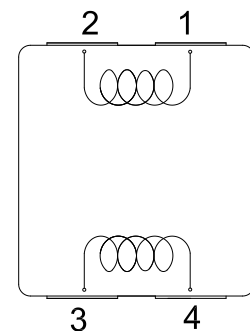
回路図
