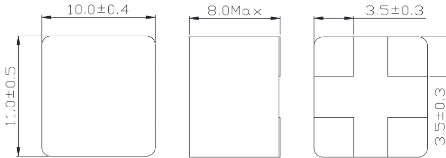
外形寸法（単位：mm）
