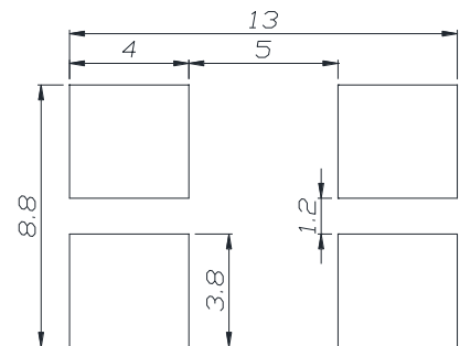
ランドパターン（単位：mm）
