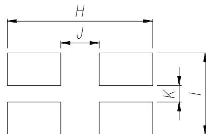
ランドパターン（単位：mm）
