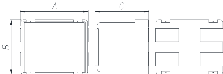
外形寸法（単位：mm）
