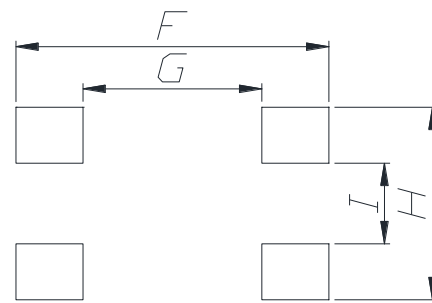
ランドパターン（単位：mm）
